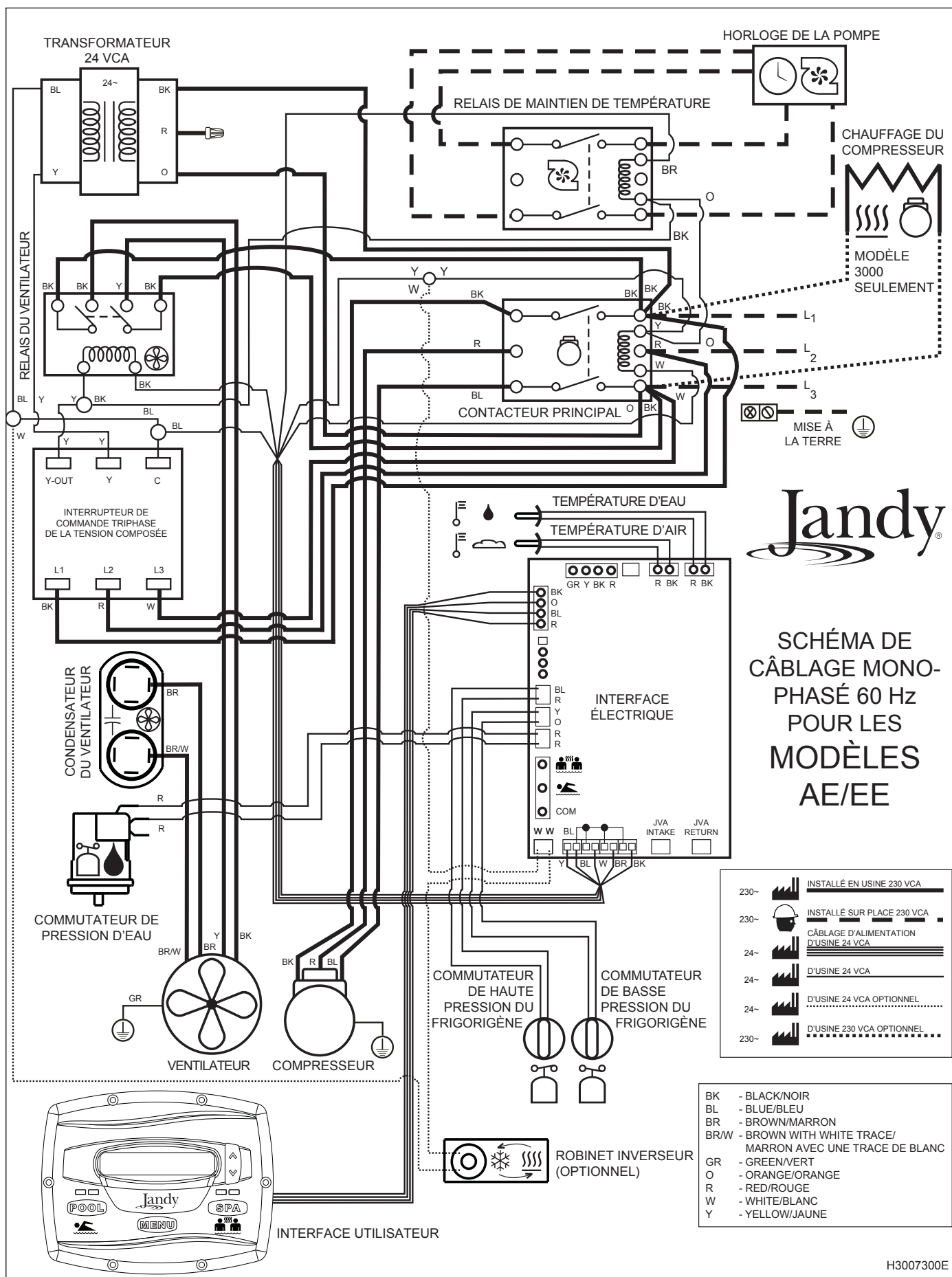
Figure 8. Diagramme de câblage électrique monophasé pour EE-Ti
