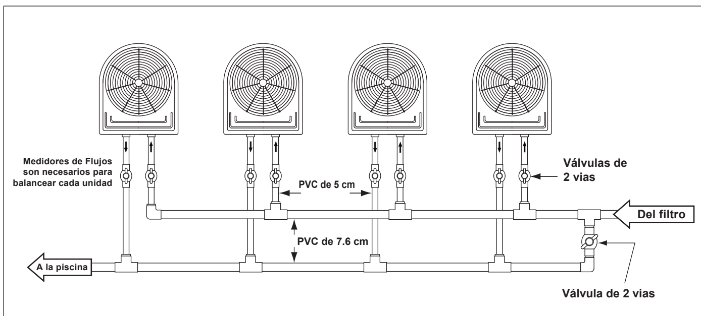
Figura 7. Hidrúlica de Cuatro Bombas de Calor
