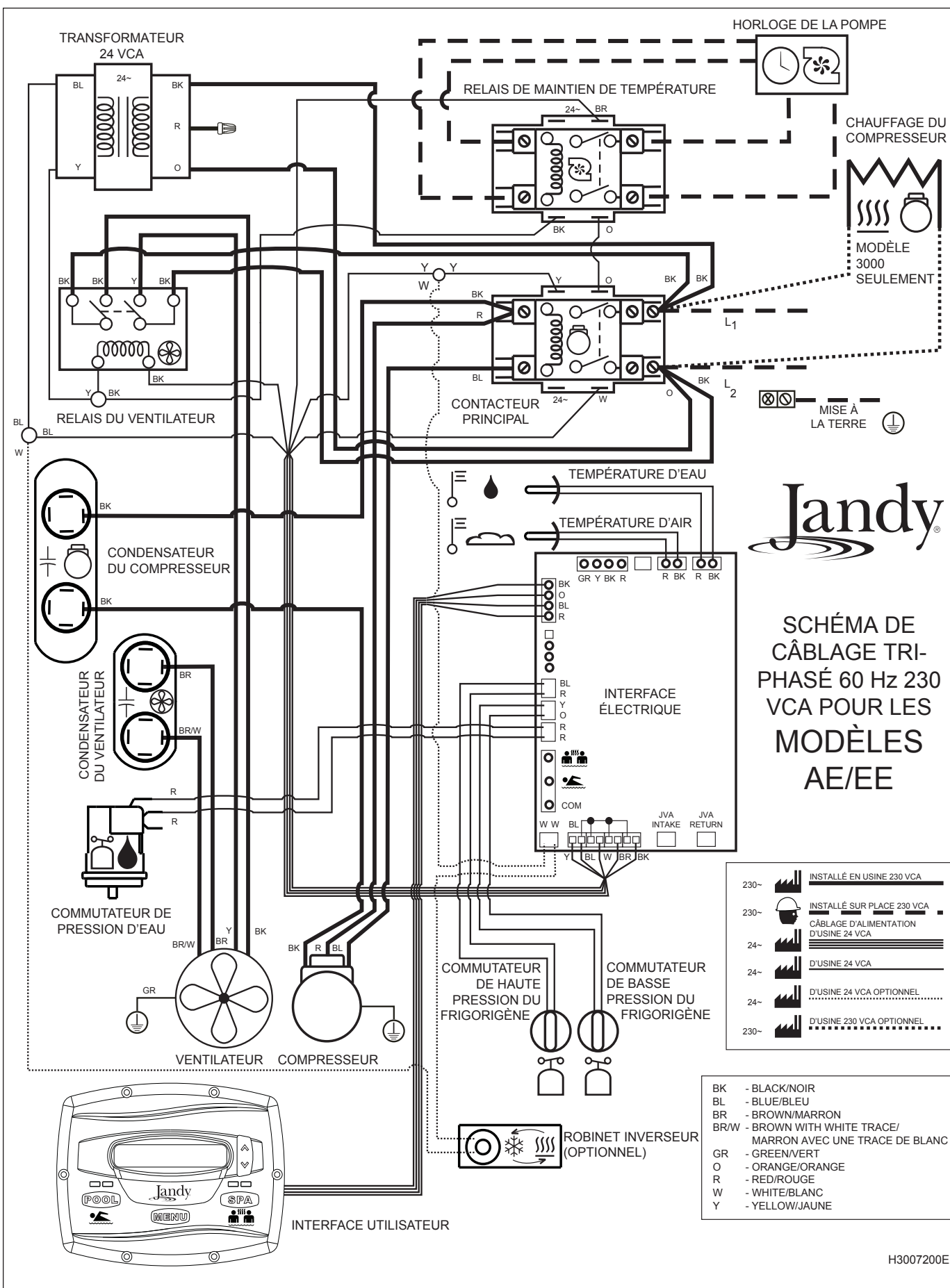
Figure 9. Diagramme de câblage électrique triphasé pour EE-Ti
