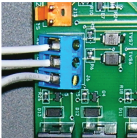
Figura 12a. Conexión a un Selector Remoto Piscina-Apagado-Spa (Conexión de 3 Cables)
