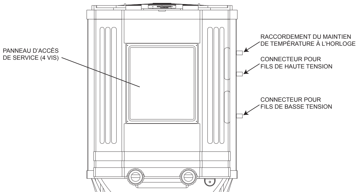
Figure 11. Vue avant de la thermopompe EE-Ti
