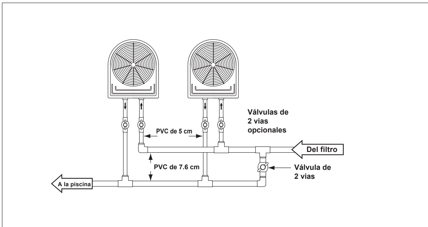
Figura 6. Hidrúlica de dos Bombas de Calor
