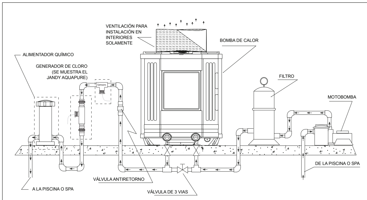
Figura 4. Hidráulica para Sistema Básico
