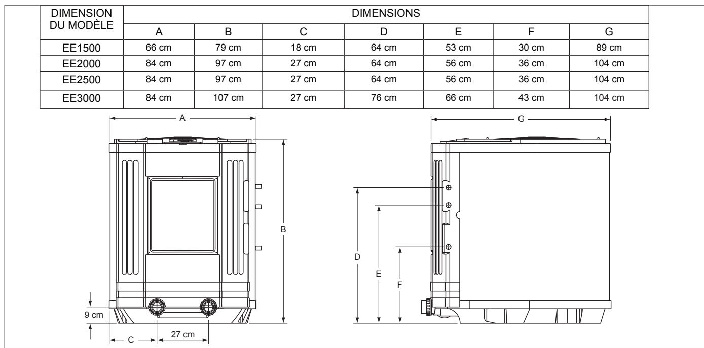
Figure 1. Dimensions des thermopompes Jandy EE-Ti
