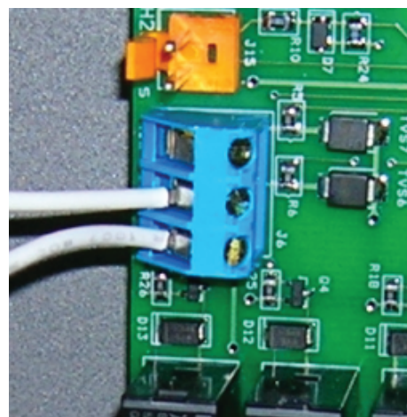
Figura 12b. Conexión a AquaLink RS o TERMOSTATO REMOTO (Conexión Bifásica)
