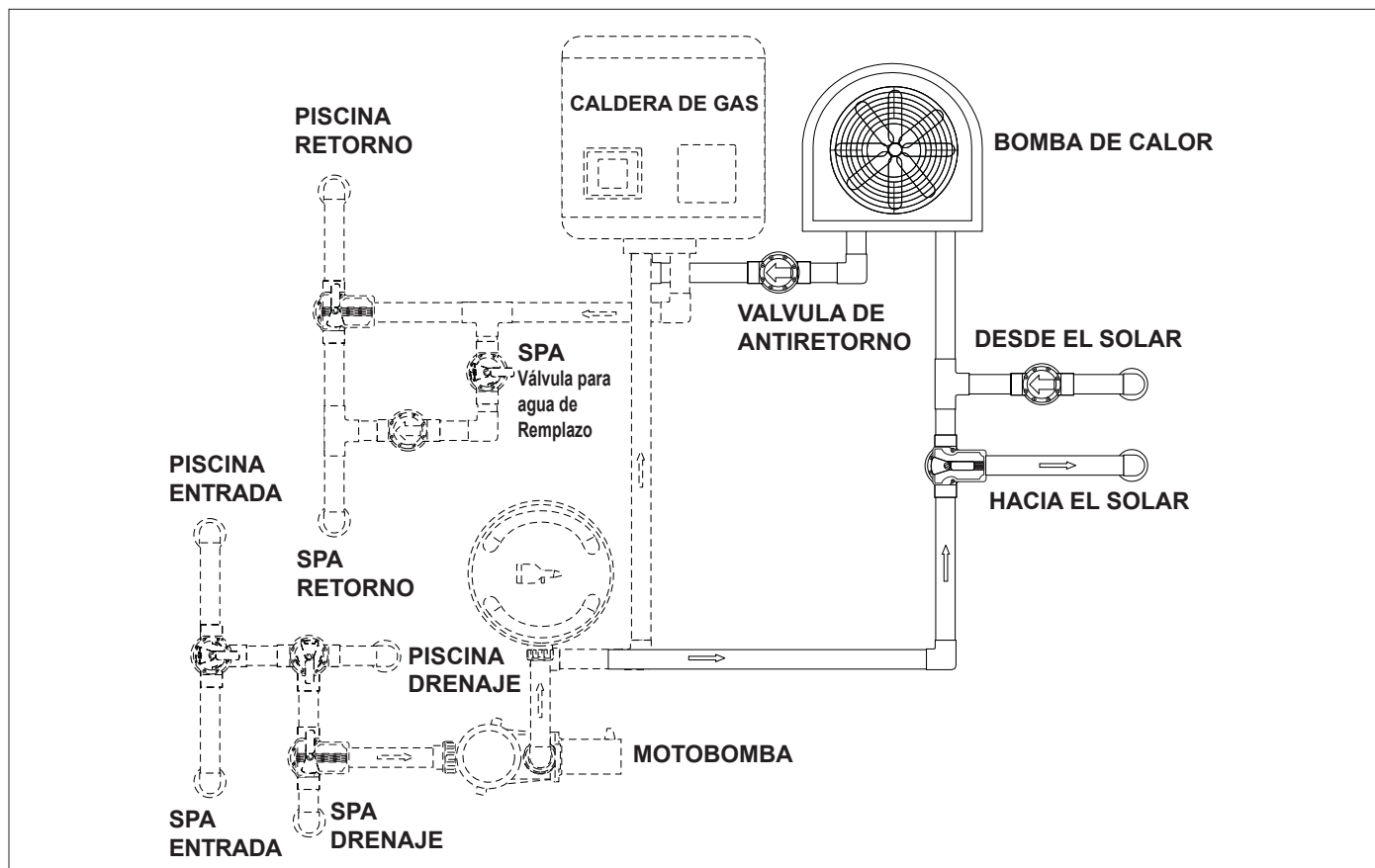
Figura 5. Hidráulica para Sistemas de Calentamiento Combinados
